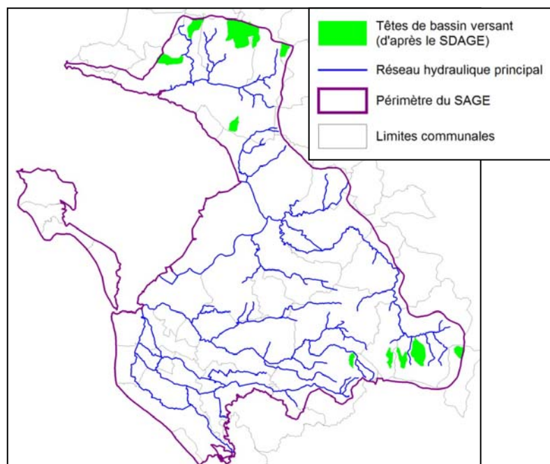
Figure 14 : Têtes de bassin versant selon la définition stricte du SDAGE Loire-Bretagne
