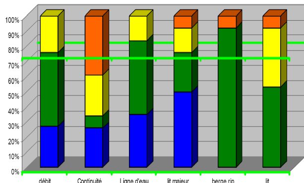
Figure 11 : Niveaux d'altération des cours d'eau du bassin versant du Falleron par compartiment (Source : SAH – 2009)
